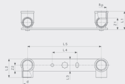
Gemini-montážní jednotka model 94476.05
