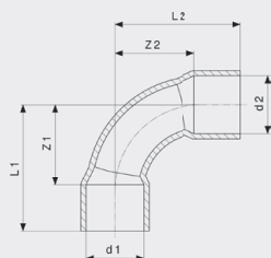
Koleno 90° - měď model 95090
