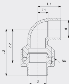
Přechodové šroubení 90° - červený bronz model 94096
