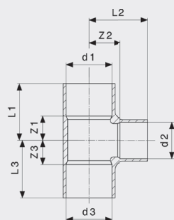
T-kus - mēd model 95130
