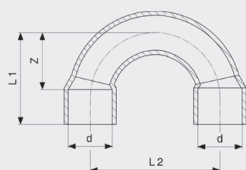
Oblouk 180° - měď model 95060
