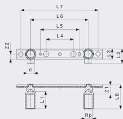
Gemini-montážní jednotka model 94476
