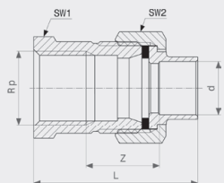
Přechodové šroubení model 94330G
