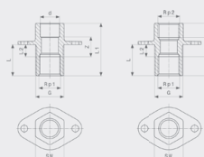
Stěnová průchodka - červený bronz model 3427
