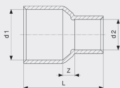
Redukční objímka - měď model 95240
