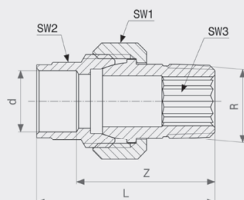
Přechodové šroubení model 94341G
