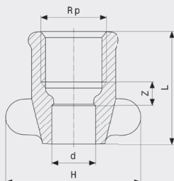
Přechodový kus - červený bronz model 94270GF
