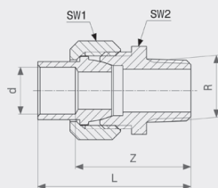
Přechodové šroubení - červený bronz model 94343G
