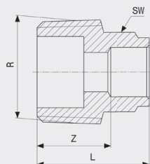
Přechodový kus - červený bronz model 94243G
