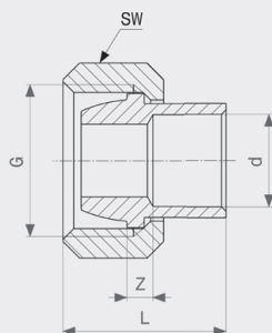
Připojovací šroubení - červený bronz model 94384G
