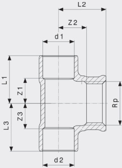
T-kus - červený bronz model 94130G
