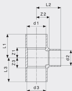
T-kus - měď model 95130
