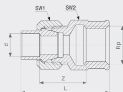
Přechodové šroubení model 94340G
