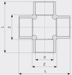
Křížová tvarovka - červený bronz model 94180
