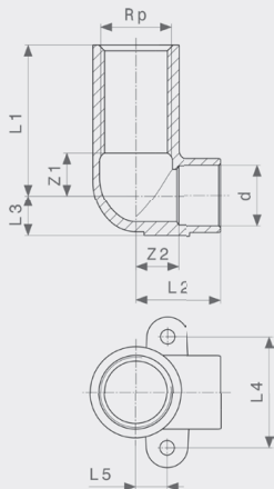
Nástěnka - červený bronz model 94472GL
