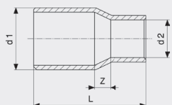
Redukce - měď model 95243
