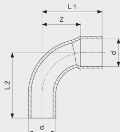
Oblouk 90° - měď model 95001A
