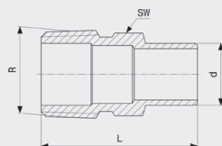
Přechodový kus - červený bronz model 94280G
