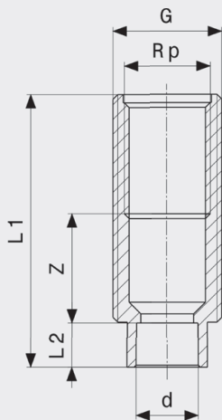
Štěnová průchodka - červený bronz model 3427.2
