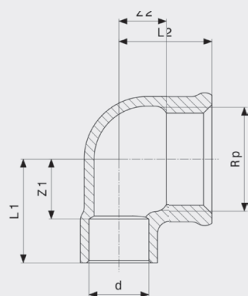
Přechodové koleno 90° - červený bronz model 94090G
