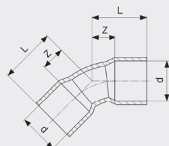
Oblouk 45° - měď model 95041
