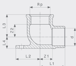
Nástěnka - červený bronz model 94471G
