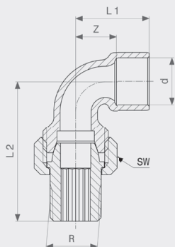
Přechodové šroubení 90° model 94098G
