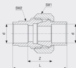
Šroubení - červený bronz model 94340
