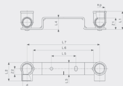
Gemini-montážní jednotka model 94476.0
