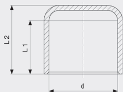
Víčko - měď model 95301
