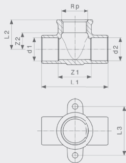
Nástěnný T-kus - červený bronz model 94490G
