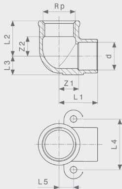
Nástěnka - červený bronz model 94472G
