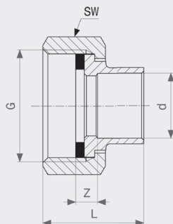
Připojovací šroubení model 94359
