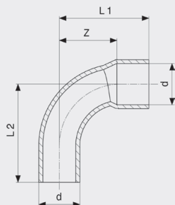
Koleno 90° - měď model 95092
