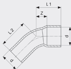
Oblouk 45° - měď model 95040
