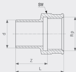
Zásuvný kus - červený bronz model 94246G
