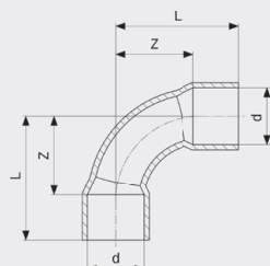
Oblouk 90° - měď model 95002A
