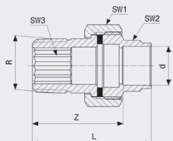
Přechodové šroubení model 94331G
