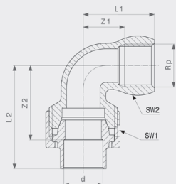
Přechodové šroubení 90° model 94096G
