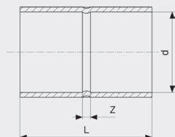
Objímka - měď model 95270
