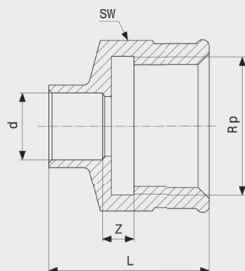
Přechodový kus - červený bronz model 94270G
