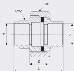
Šroubení - červený bronz model 94330
